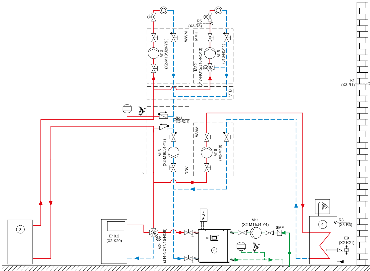
Schemat hydrauliczny 1
