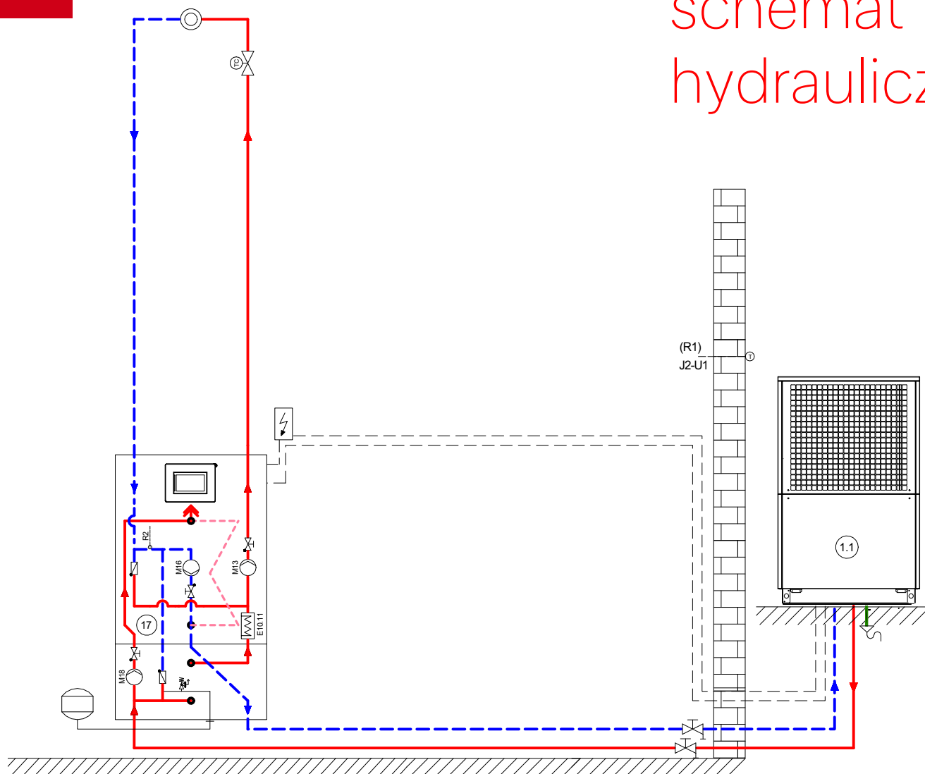
Schemat hydrauliczny 1
