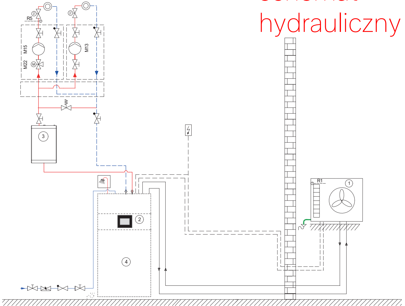
Schemat hydrauliczny 2
