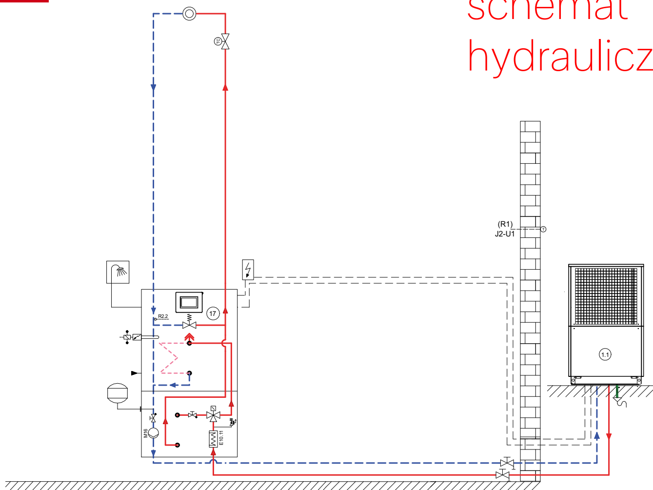
Schemat hydrauliczny 1
