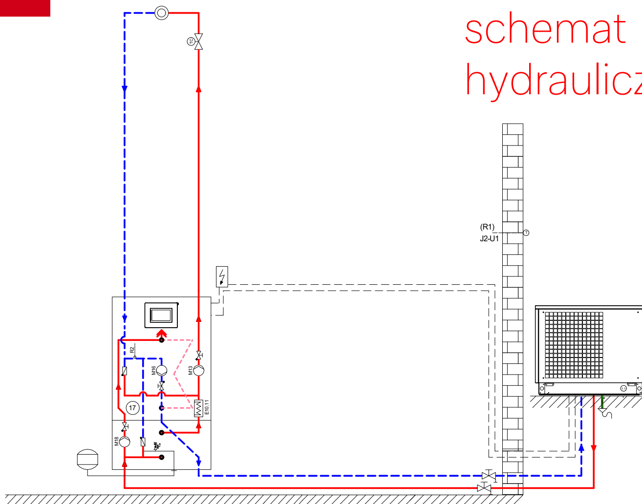
Schemat hydrauliczny 1
