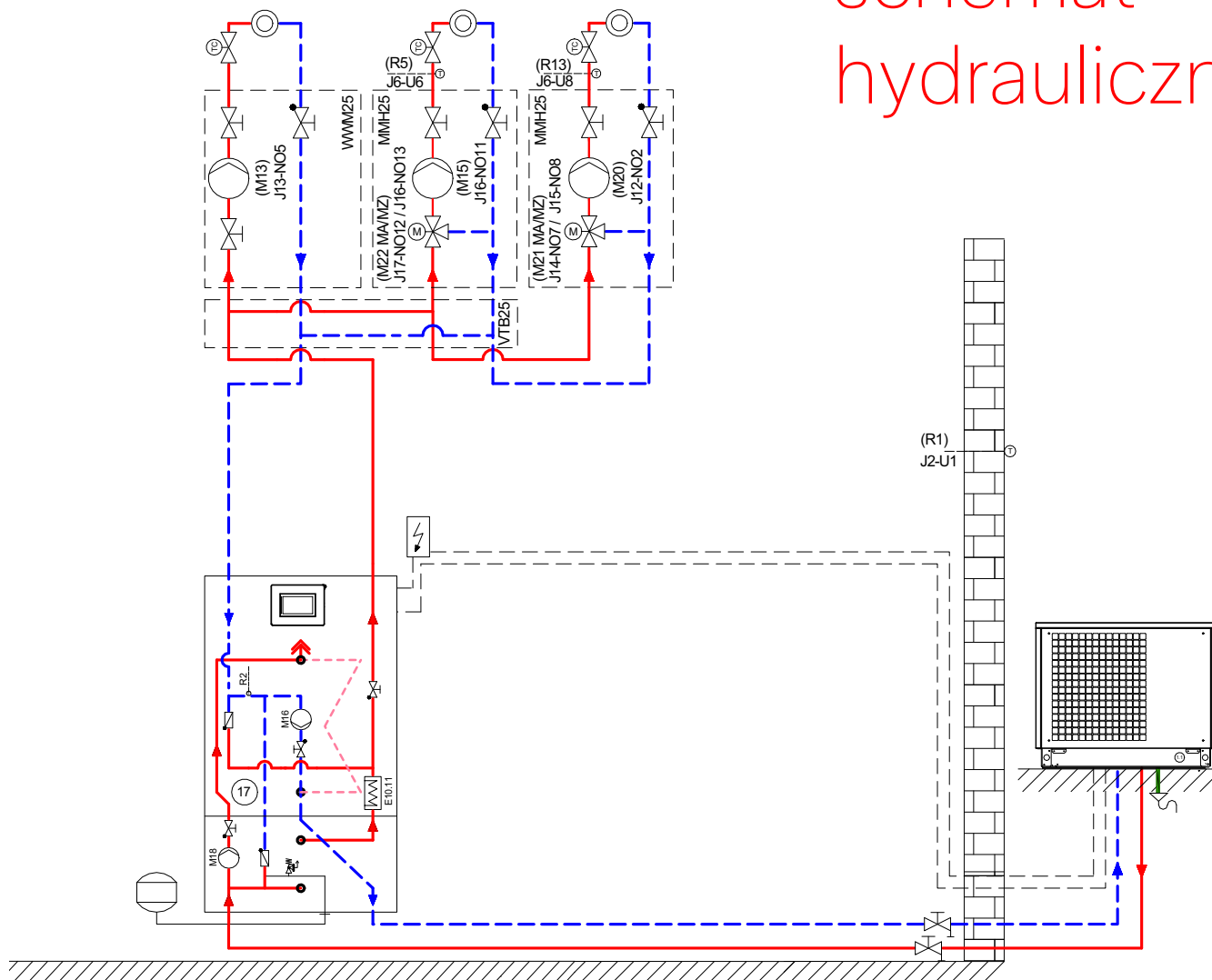
Schemat hydrauliczny 2
