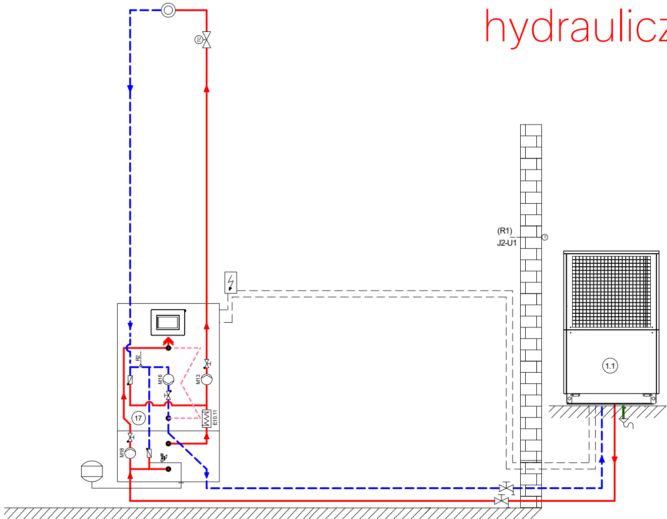
Schemat hydrauliczny 1
