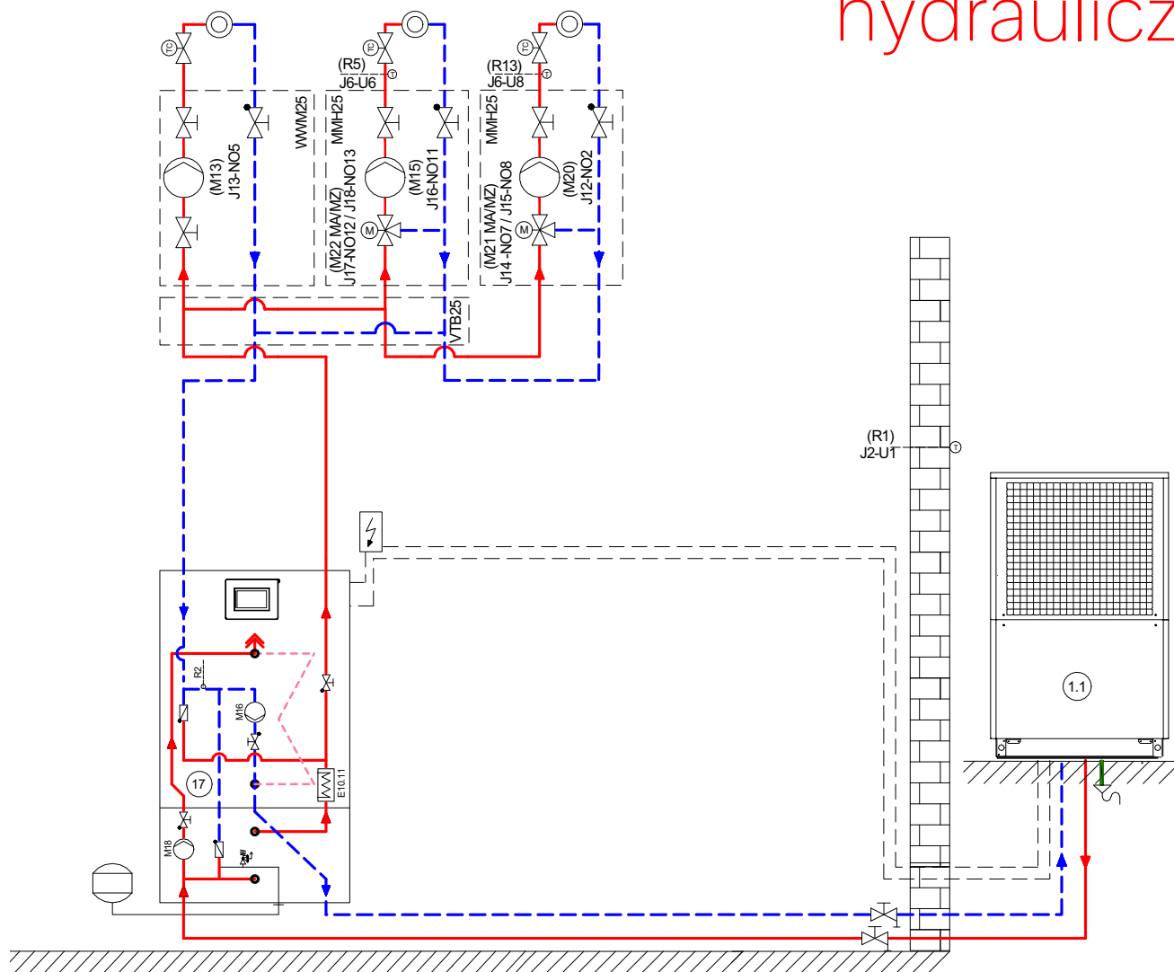
Schemat hydrauliczny 2
