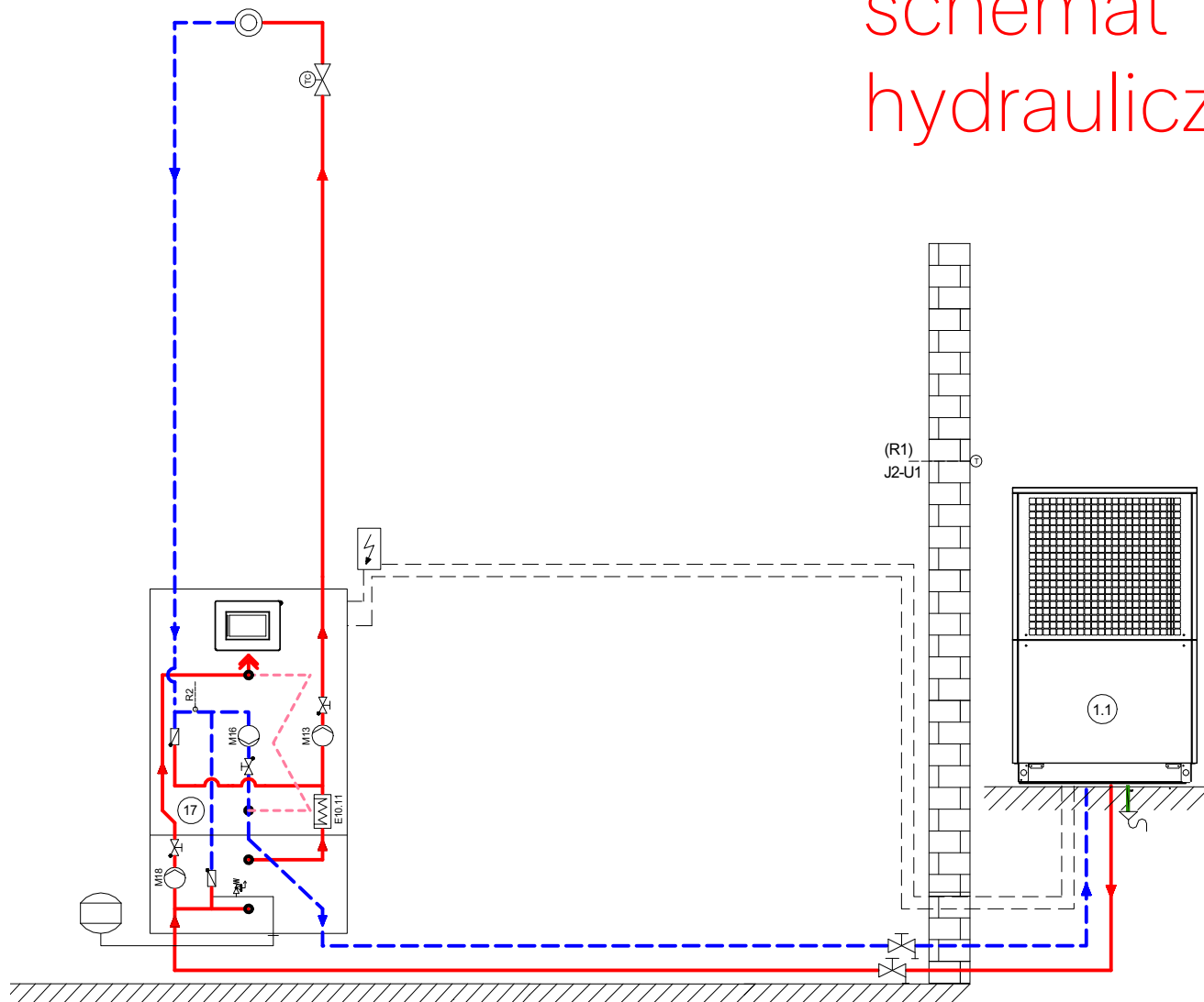
Schemat hydrauliczny 1
