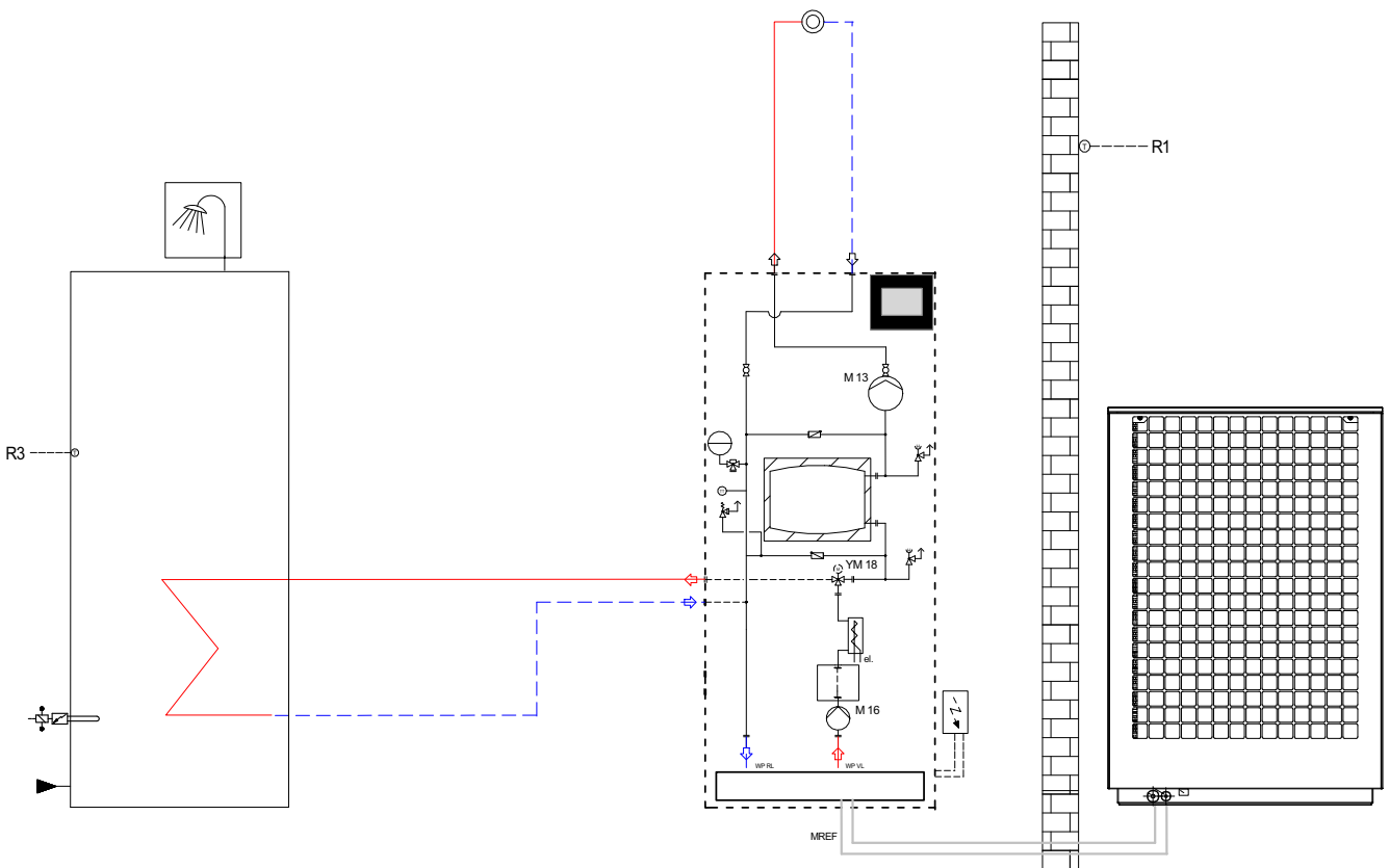
Schemat hydrauliczny 2
