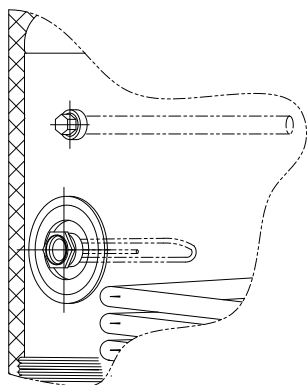
Rys. 8.1: Anoda w systemie ogrzewania elektrycznego
