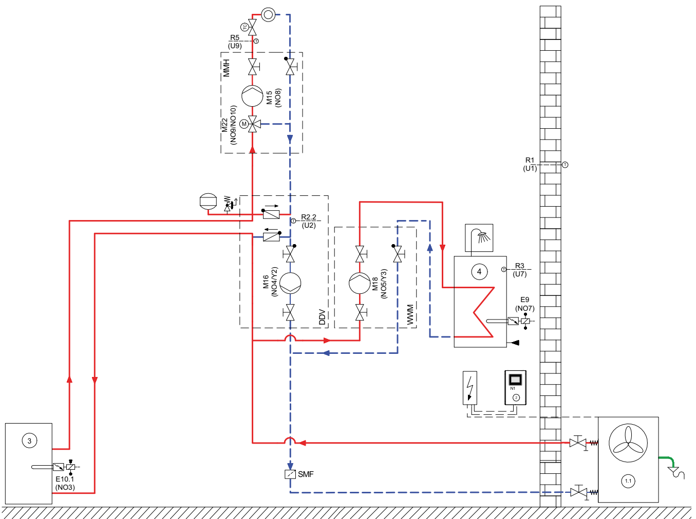
Schemat hydrauliczny 2
