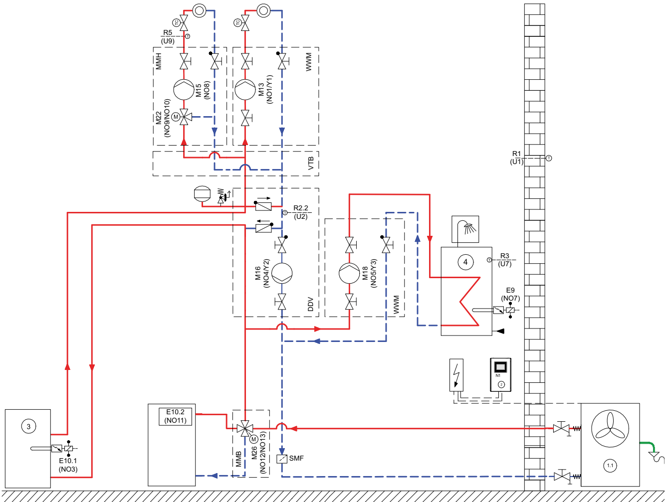
Schemat hydrauliczny 1
