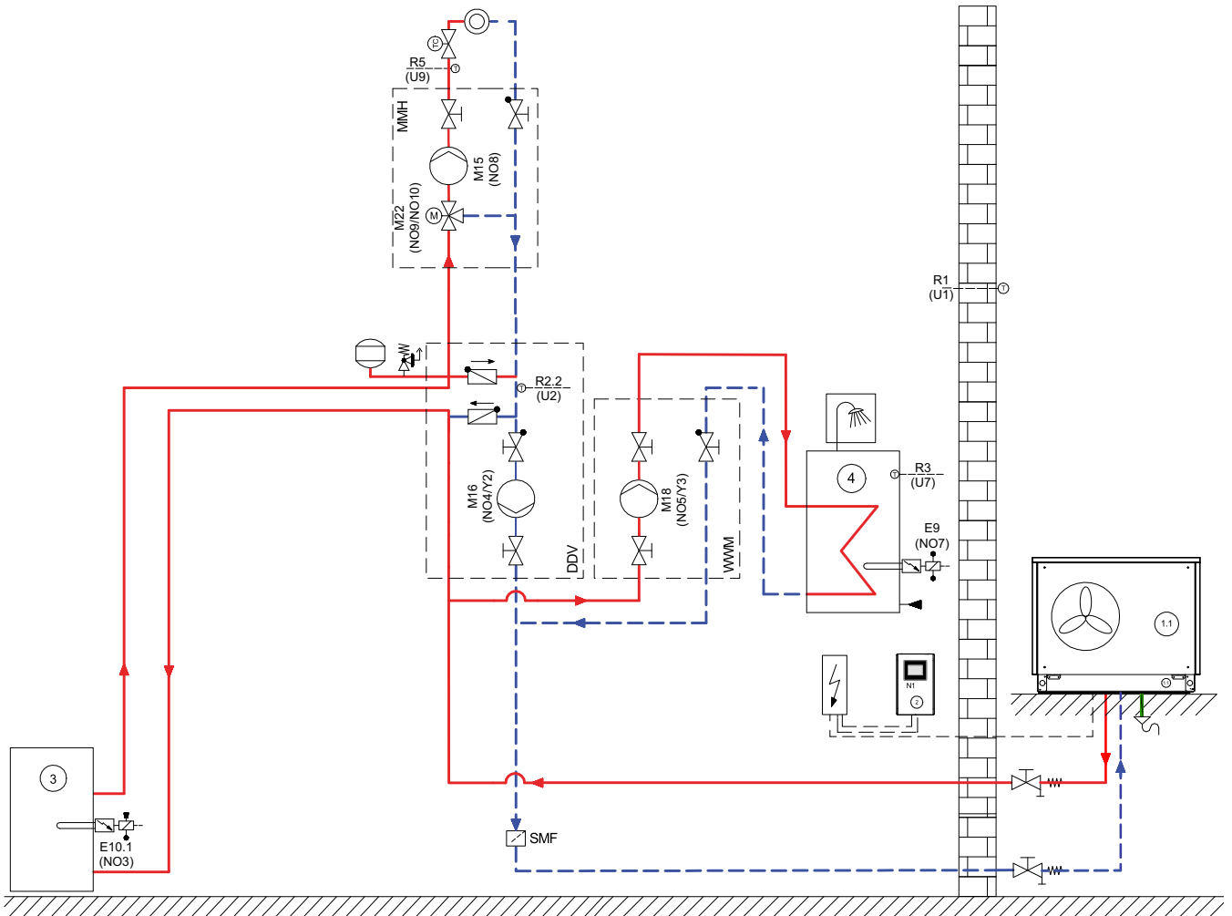
Schemat hydrauliczny 2
