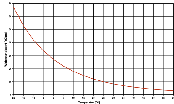
Abb. 7.2: Fühlerkennlinie NTC 10
