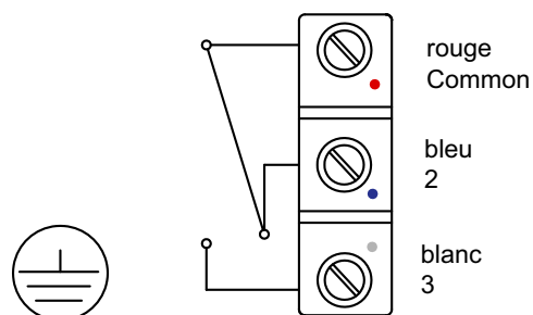
Fig. 3.2: Schéma électrique
