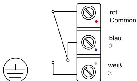
Abb. 3.2: Anschlussplan
