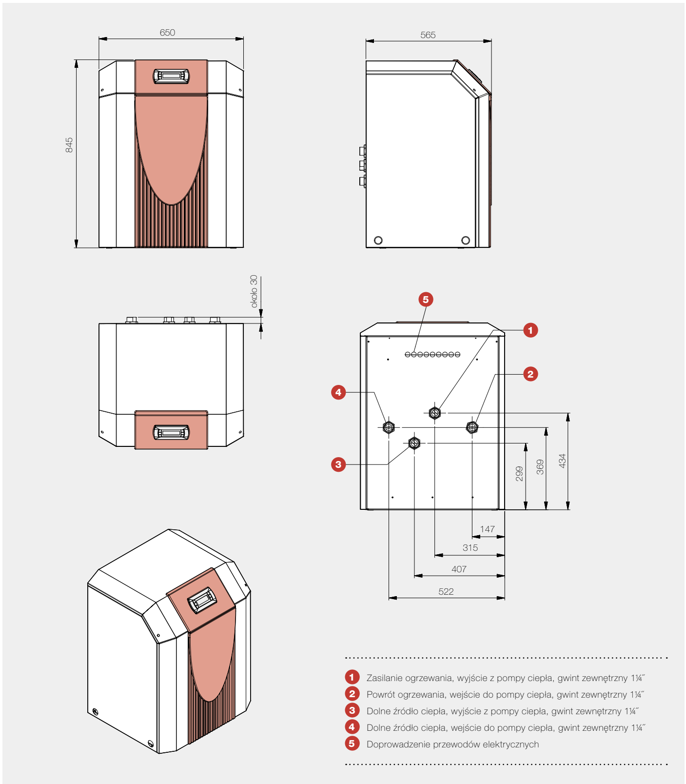
Rysunek wymiarowy
