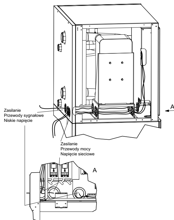
Rys. 7.3: Wpust kablowy do rozdzielni
