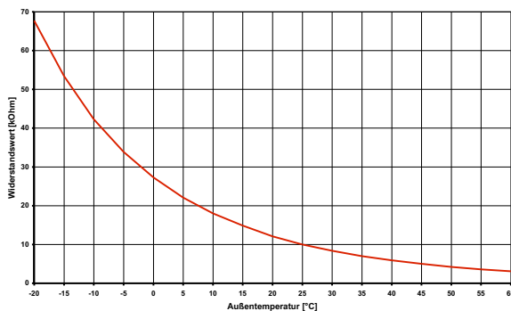
Abb. 7.2: Fühlerkennlinie NTC-10
