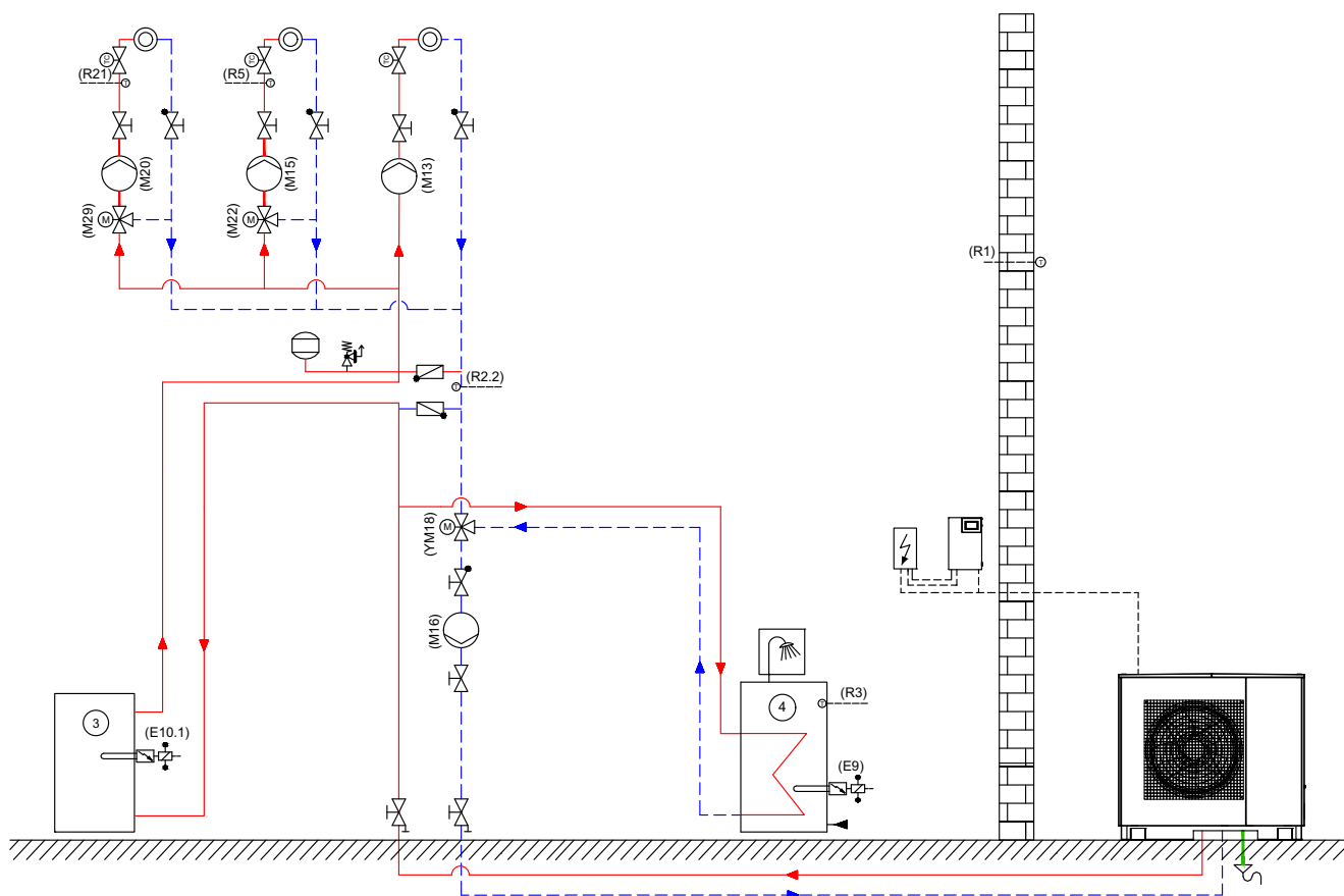
schemat hydrauliczny 1
