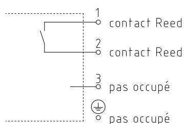
Figure 1: Schéma électrique
