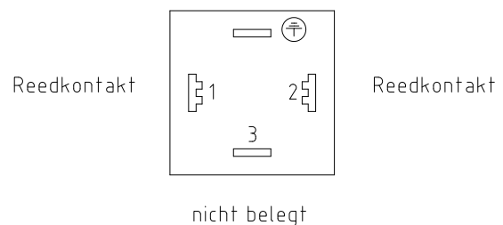
Bild 2: Anschlußplan
