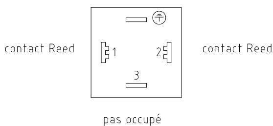
Figure 2: Schéma électrique
