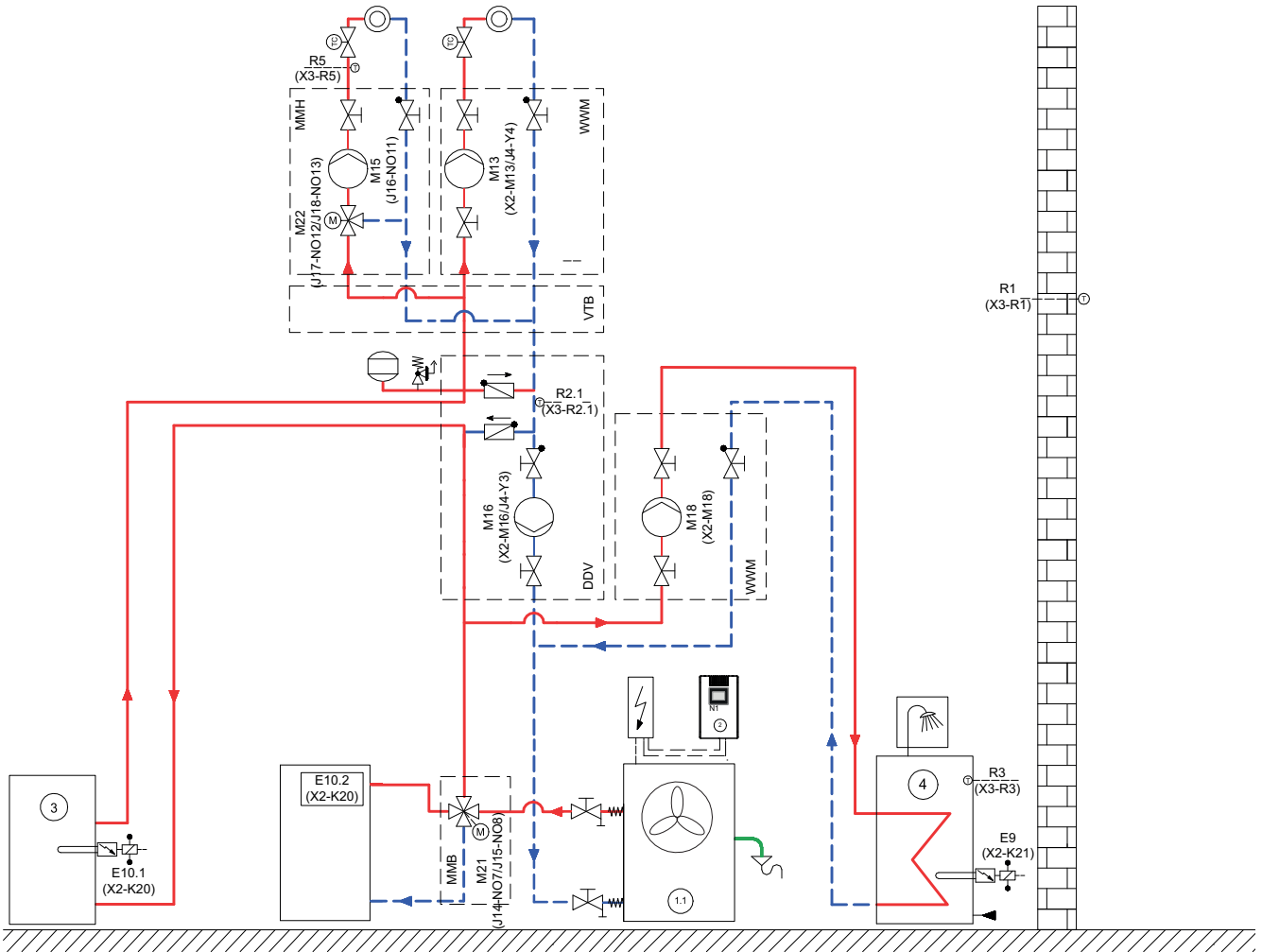
Schemat hydrauliczny 1
