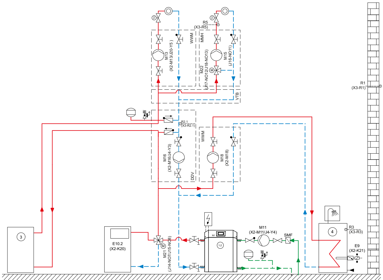
Schemat hydrauliczny 1
