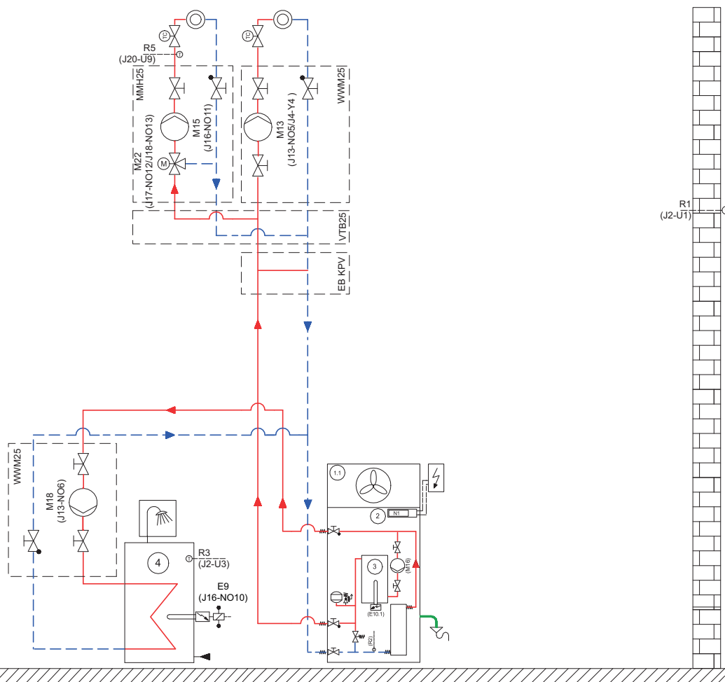
Schemat hydrauliczny 1
