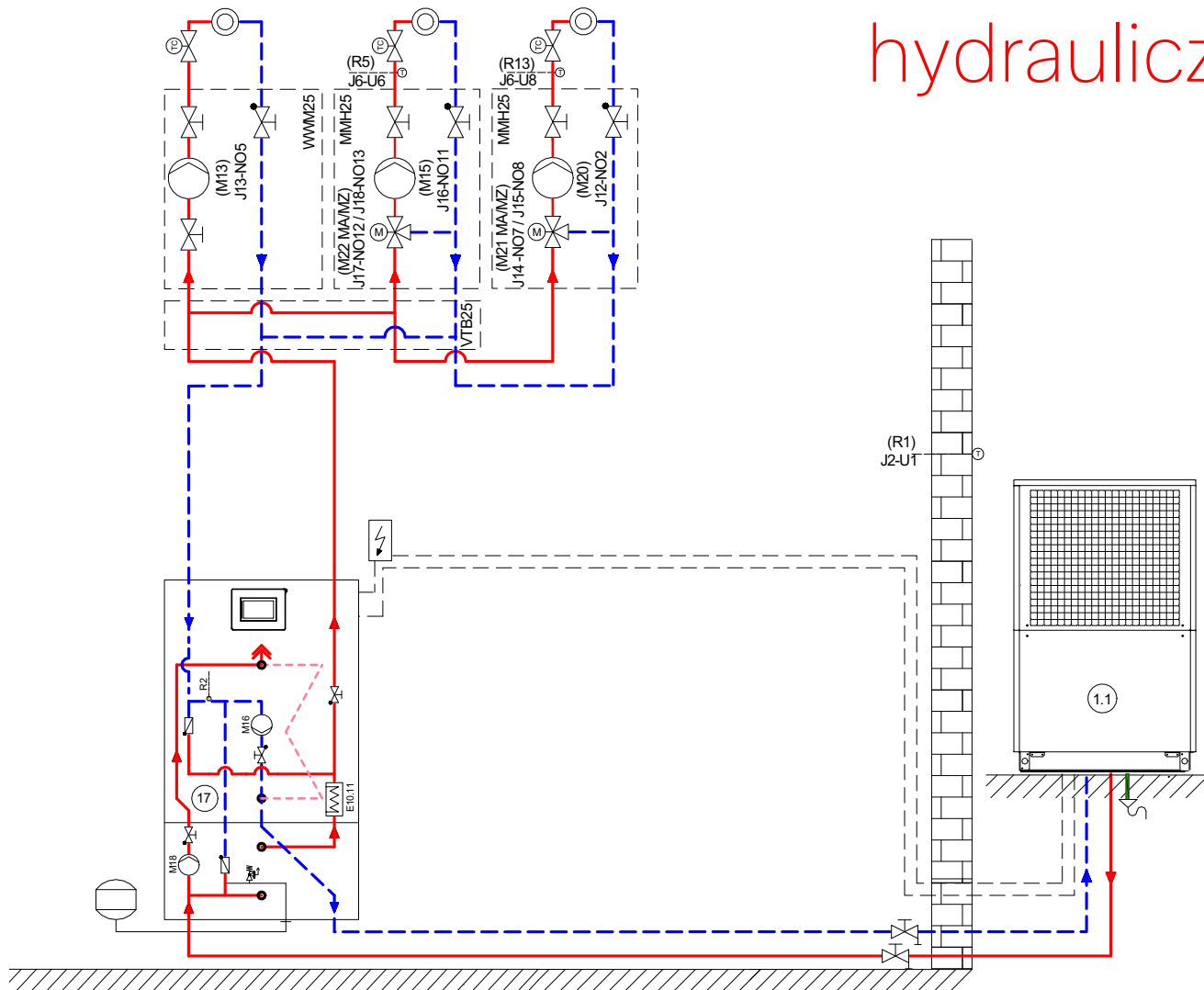
Schemat hydrauliczny 2
