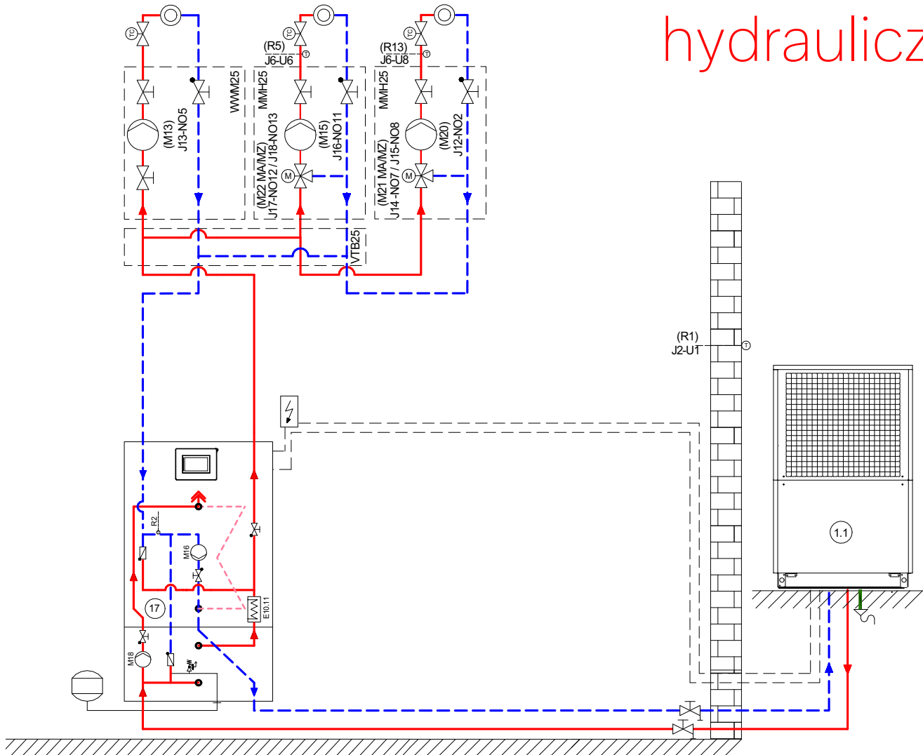
Schemat hydrauliczny 2
