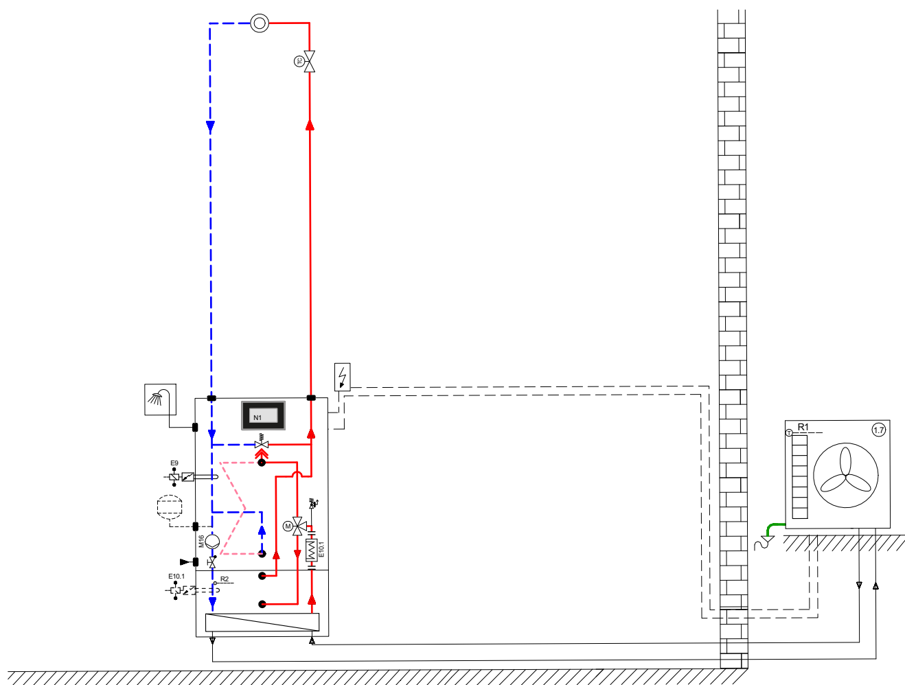
Schemat hydrauliczny 1
