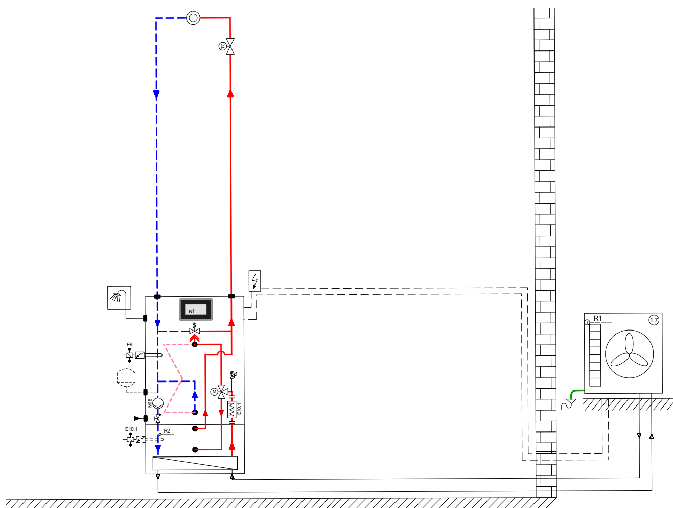
Schemat hydrauliczny 1
