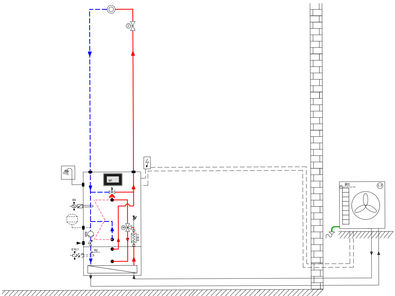
Schemat hydrauliczny 1
