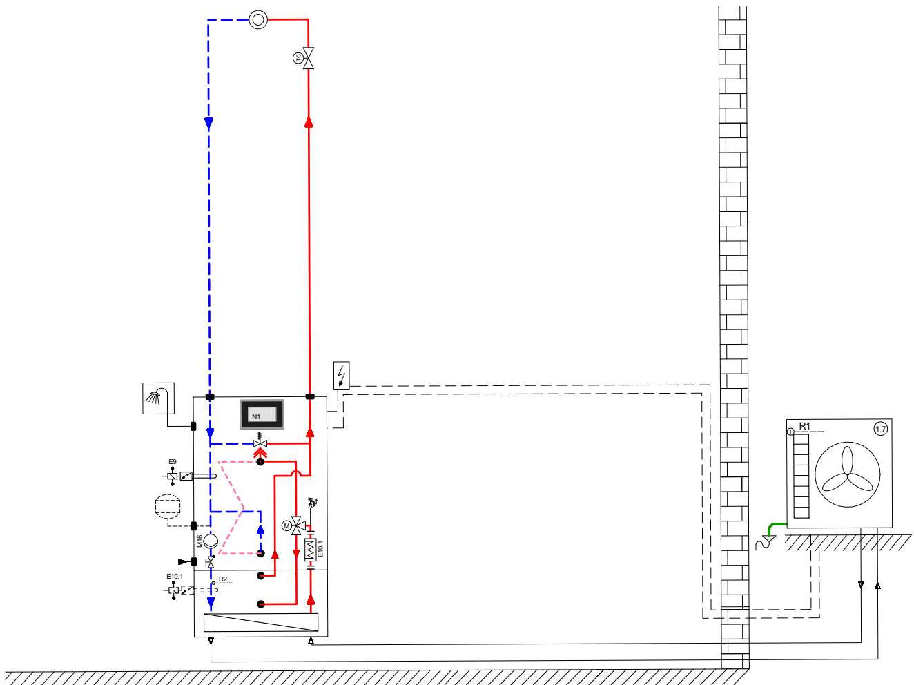
Schemat hydrauliczny 1
