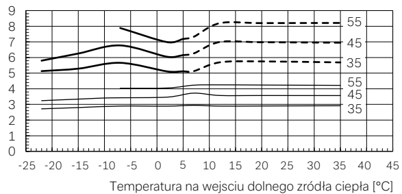
Pobór mocy elektrycznej z udziałem pompy i wentylatora wg EN 14511 [kW]
