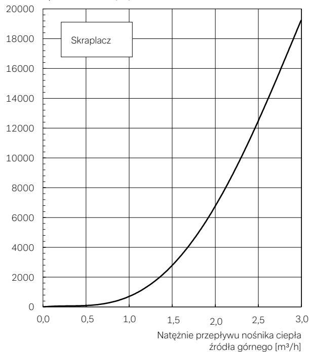
Spadek ciśnienia [Pa]
