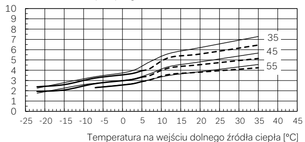
COP z udziałem pomp wg EN 14511 w [-]
